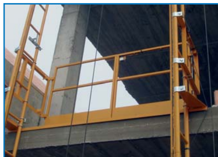
Puerta en planta Floor door
