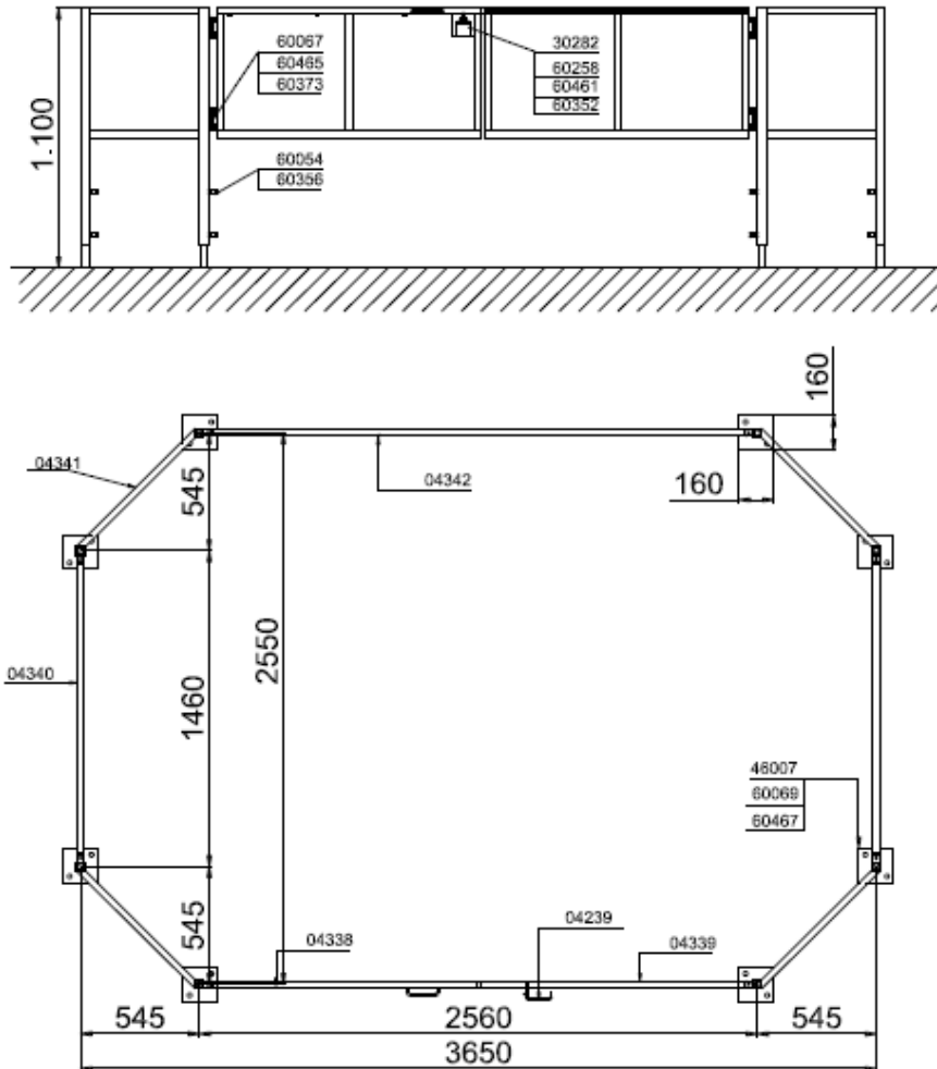
Plano 9 - CERRAMIENTO DE BASE
