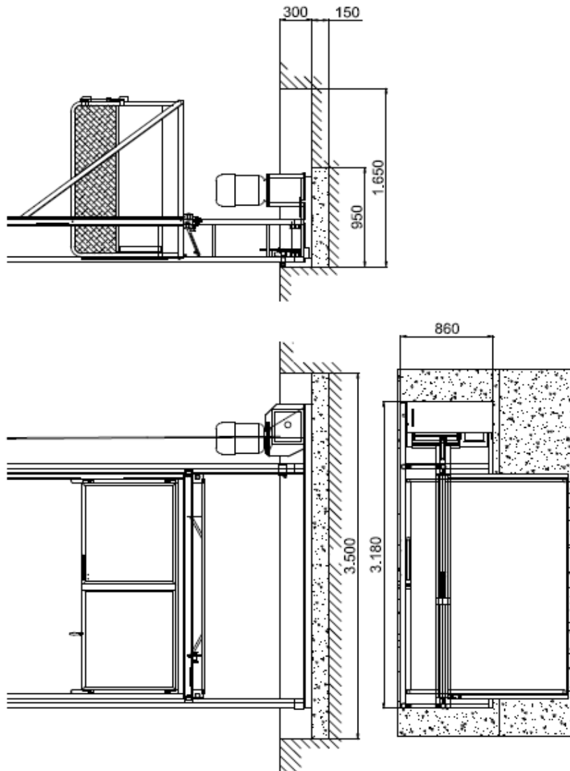
Plano 11 - CIMENTACIÓN CON FOSO
